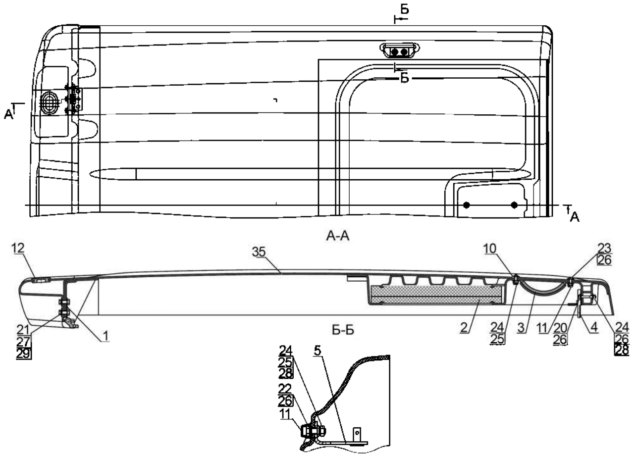
Рис.67.3. Крыша
