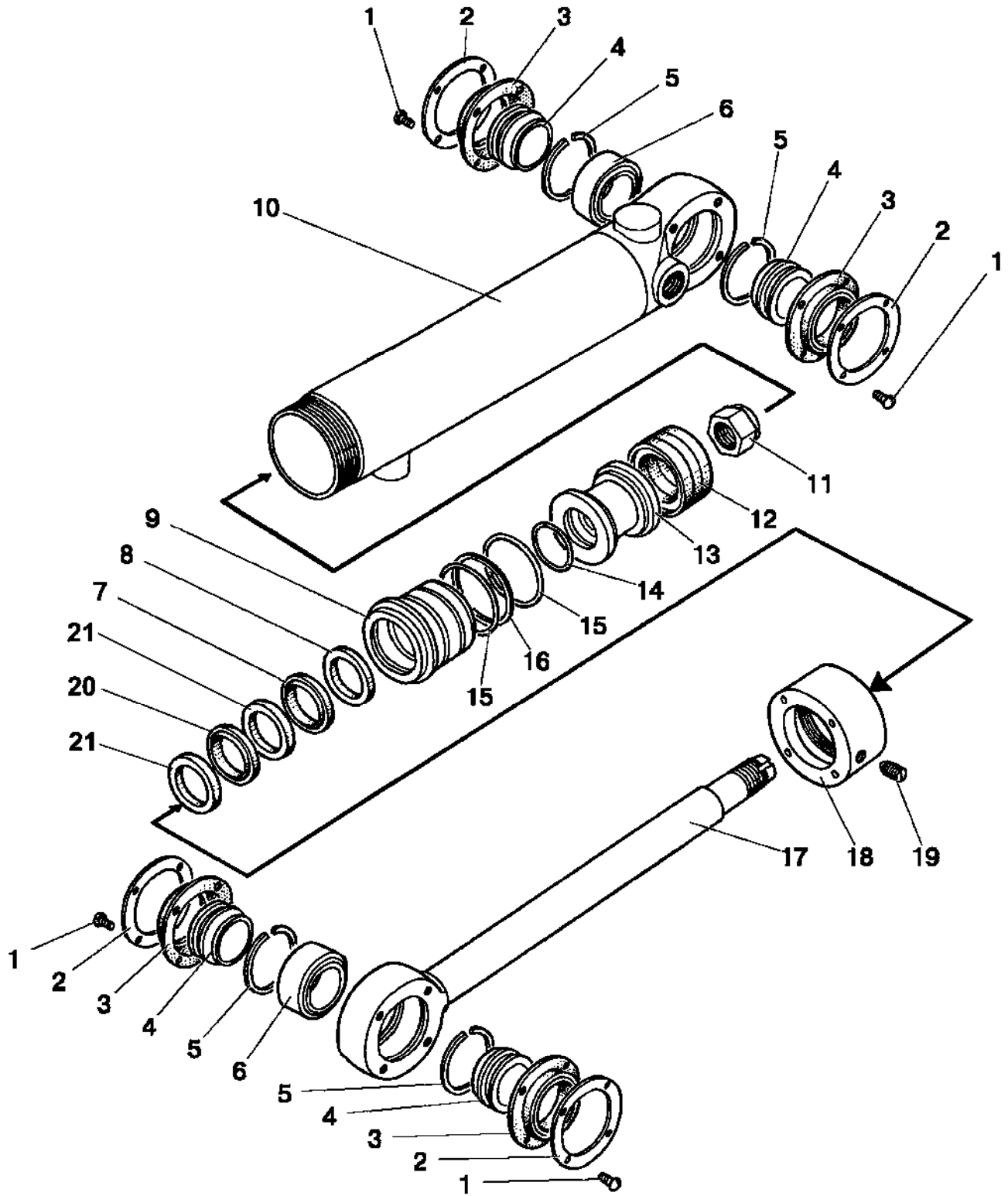
Рис. 34.6. Гидроцилиндр Ц63
