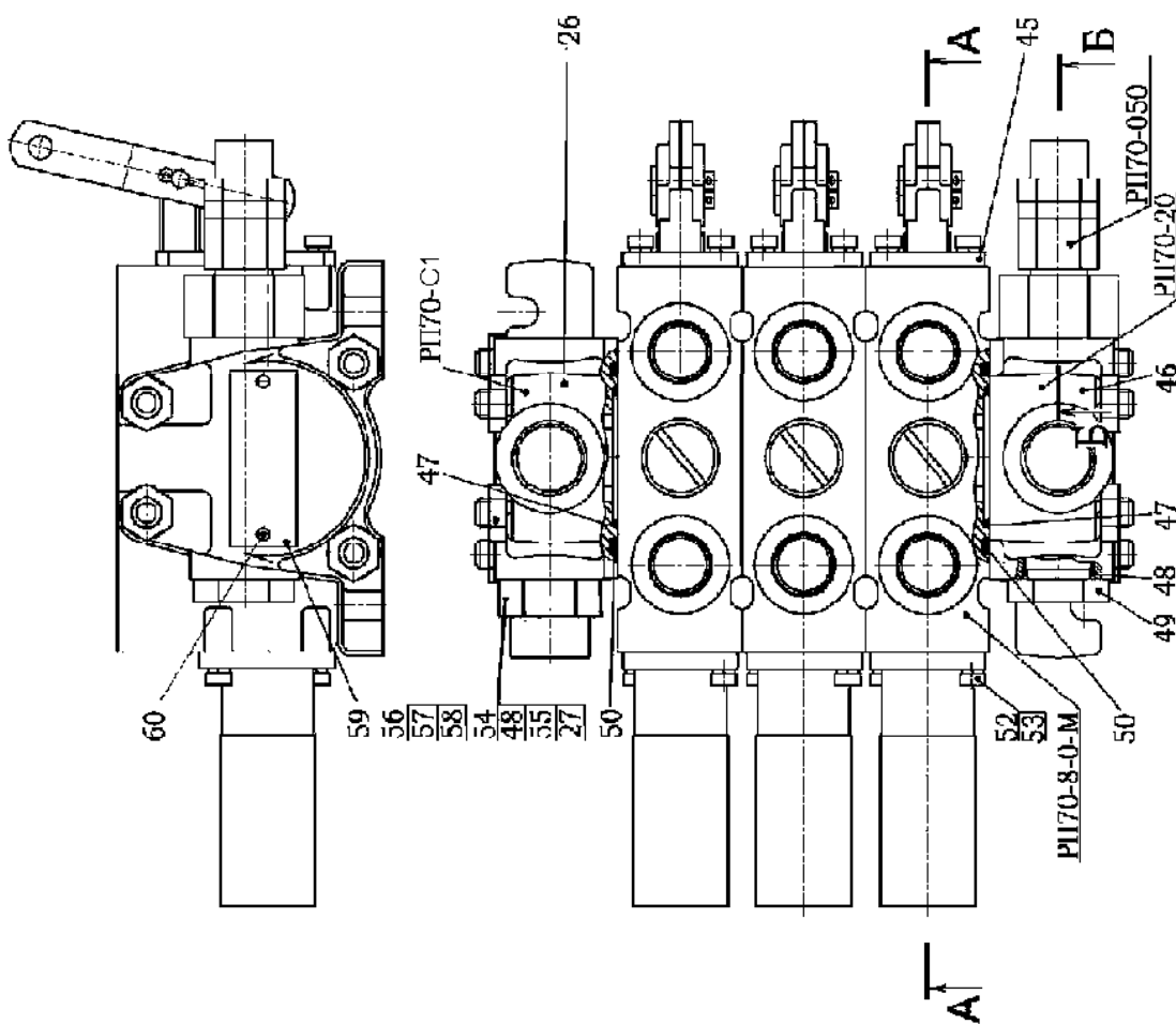
Рис.46.10. Гидрораспределитель РП70
