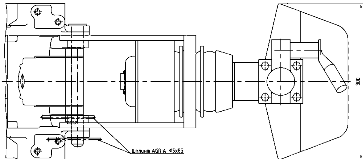
Рис. 28.2. Устройство буксирное
