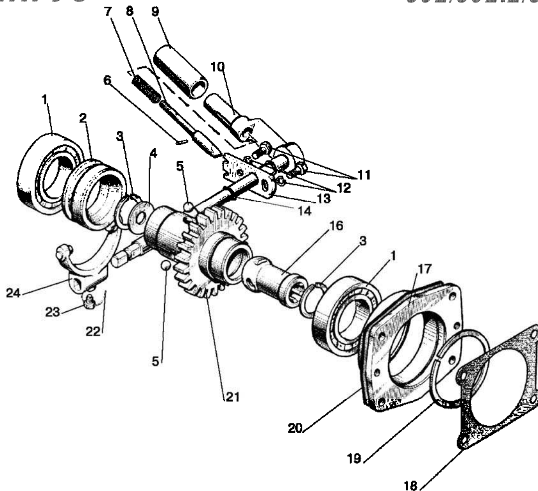
Рис.46.12. Привод насоса
