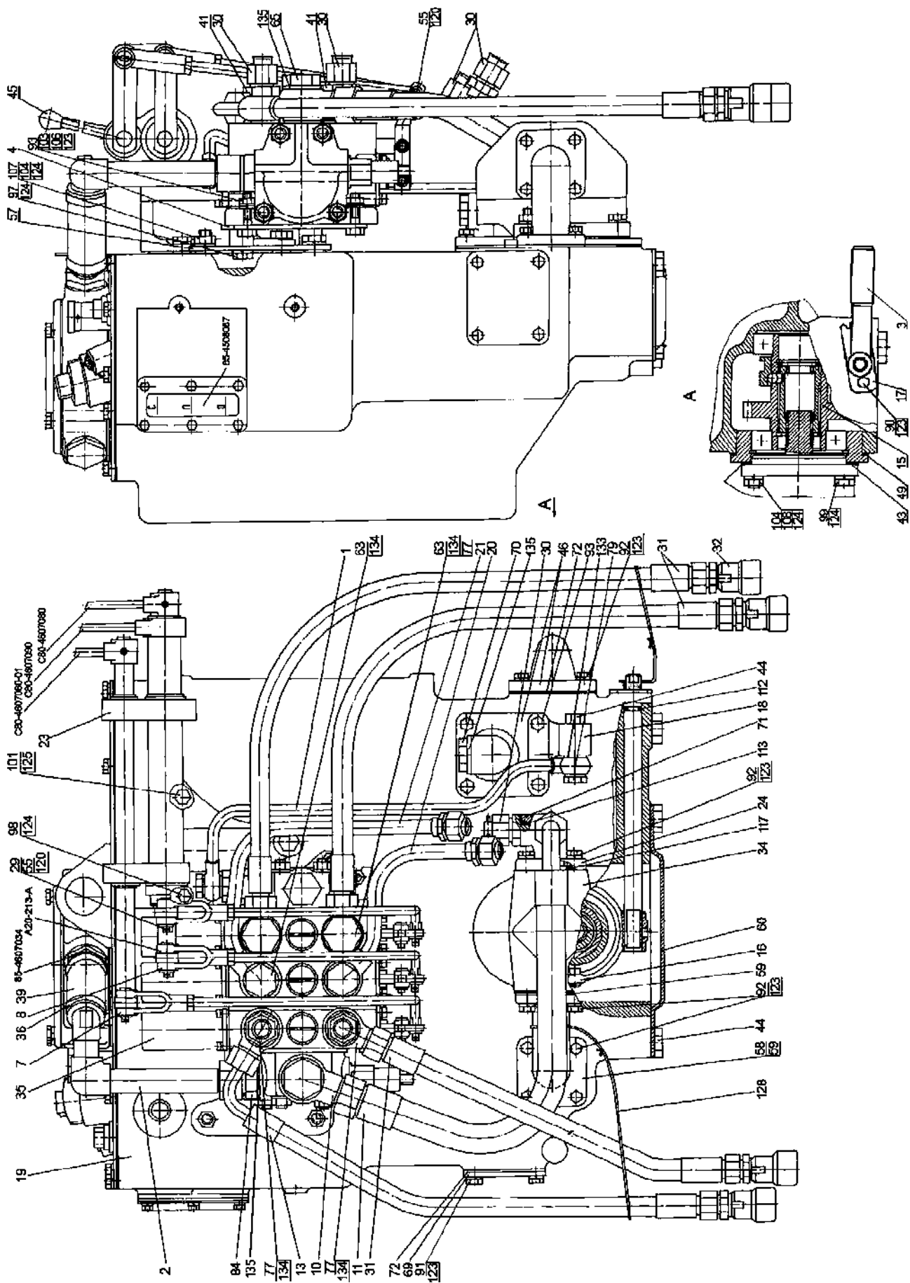
Рис.46.8. Корпус гидросистемы P85-460015-01
