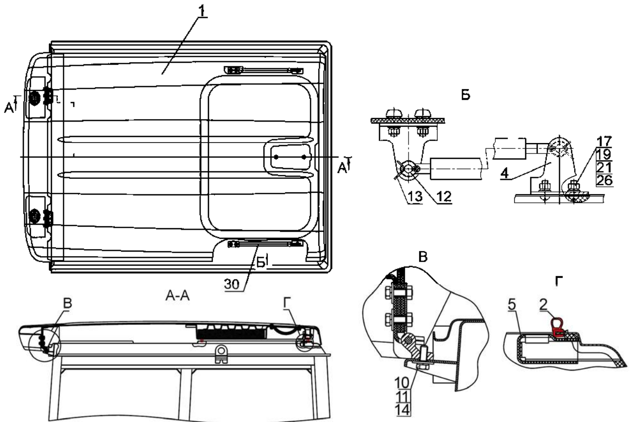
Рис.67.4. Крыша
