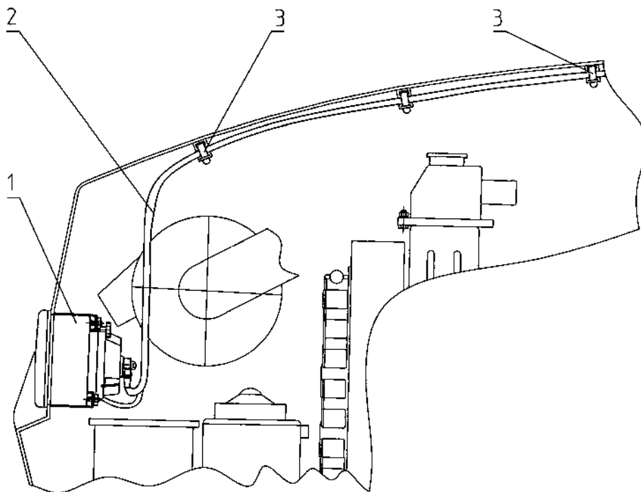
Рис.37.4. Установка фар дорожных (921-370020-01)
